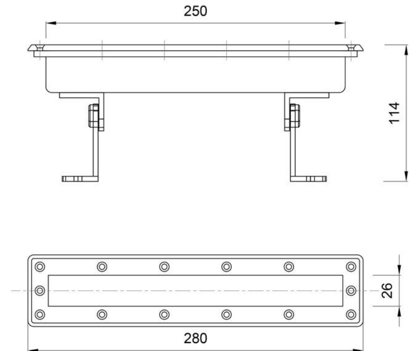
Чертёж изделия
