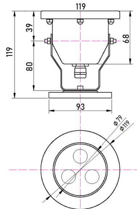
Чертёж изделия
